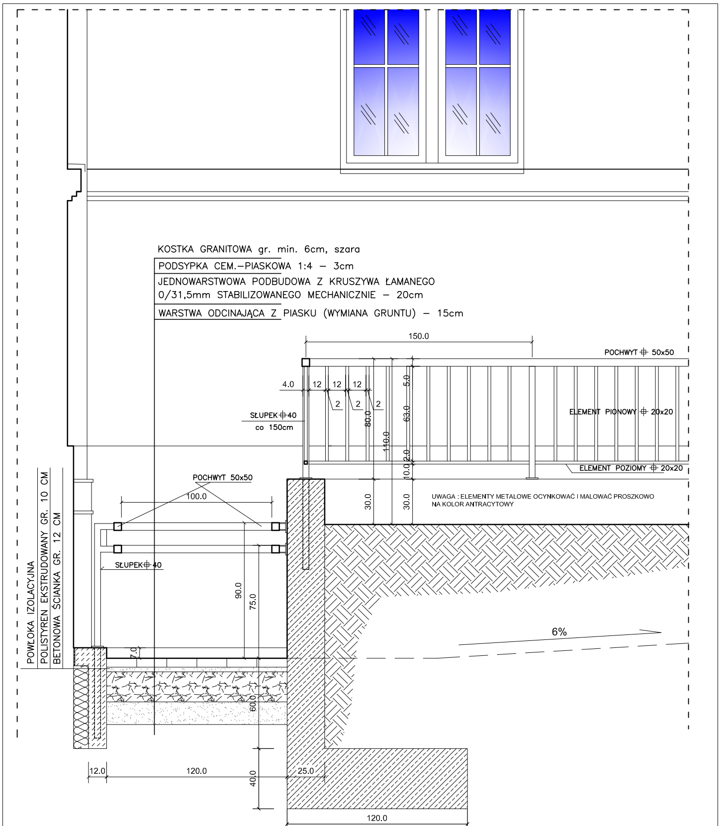
Przekrój D-D Skala 1:25
