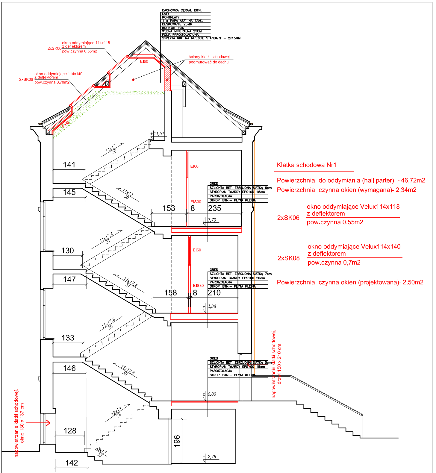
Przekrój B-B Skala 1:100
