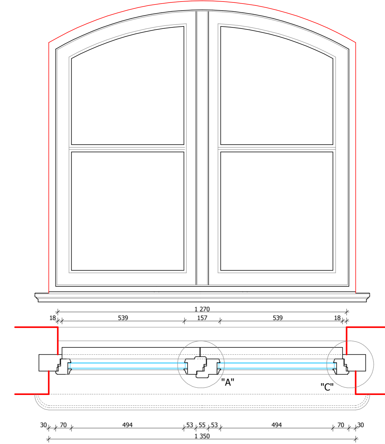
przekrój poziomy
