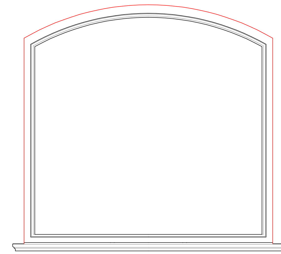
widok oboknia od wewnątrz skala 1:10
