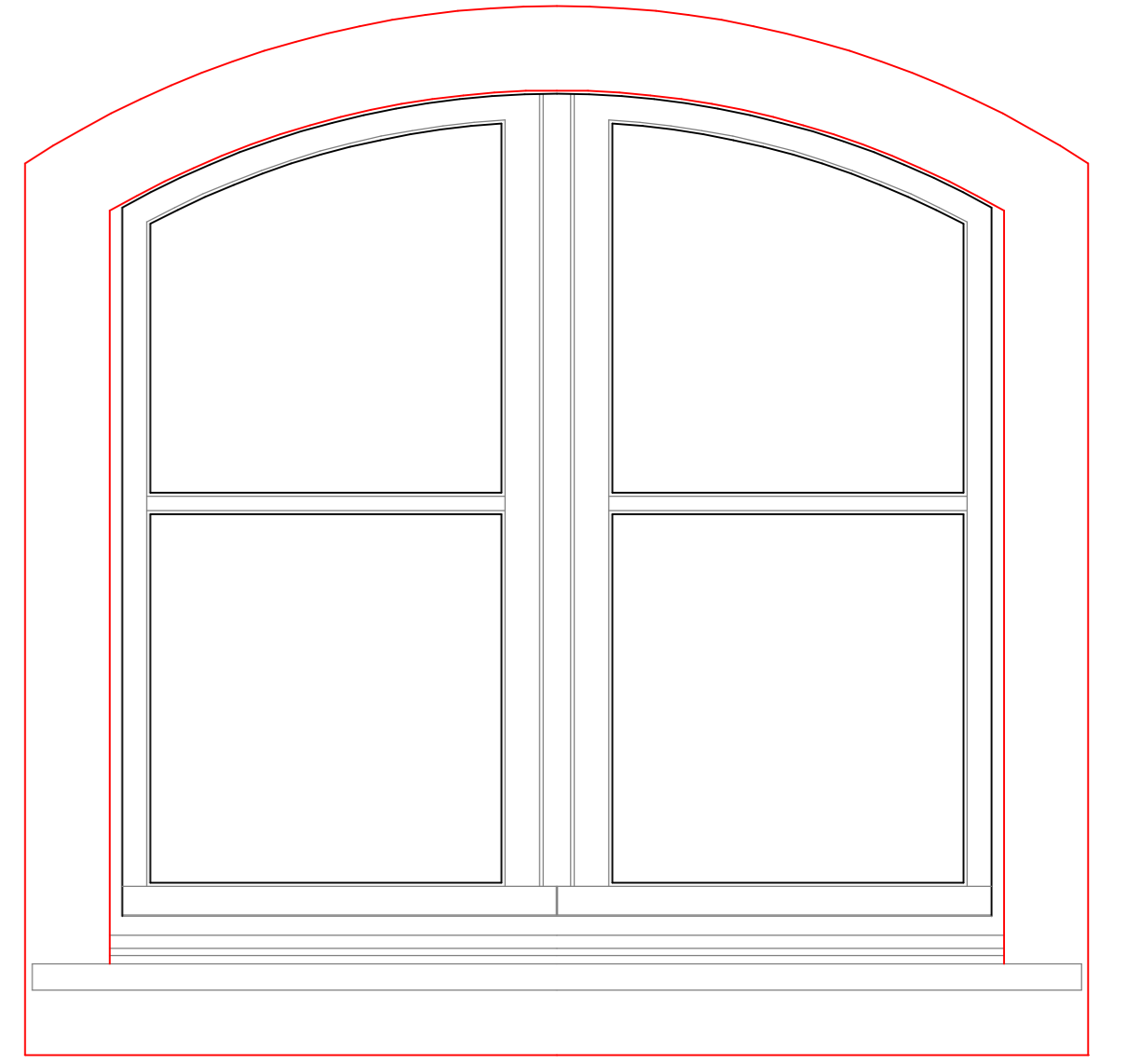
widok z zewnątrz skala 1:10
