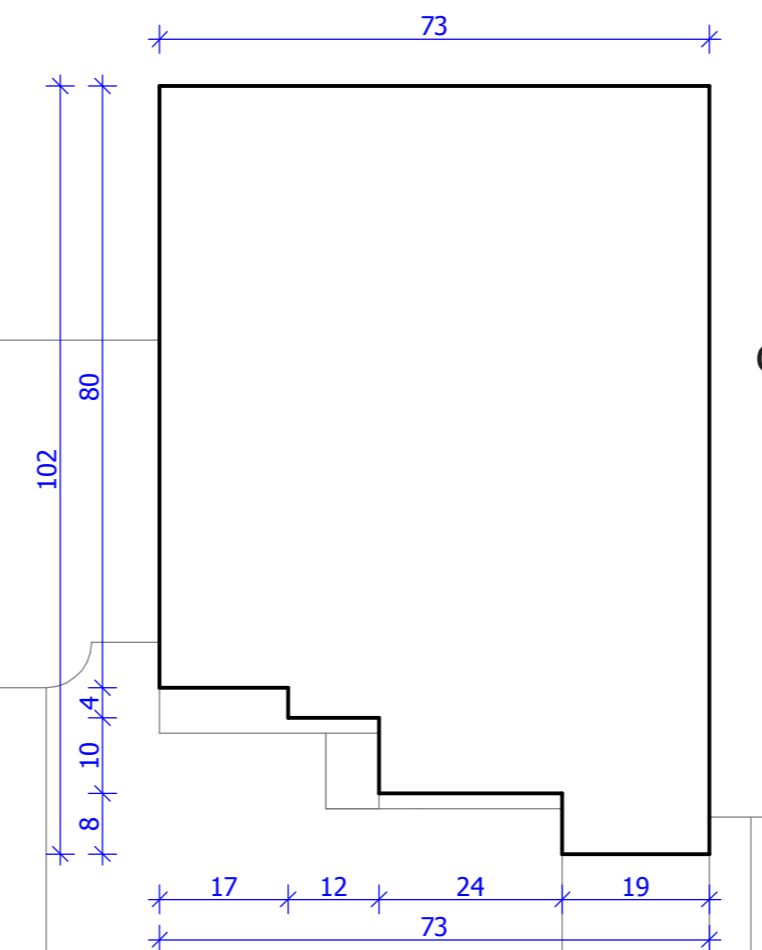
widok wew. oboknia od skala 1:10
