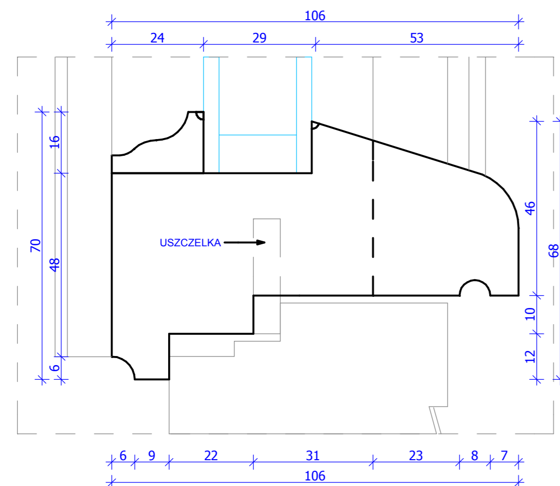
detal "D" skala 1:1
