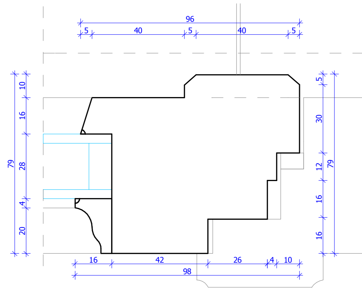
detal "A" skala 1:1
