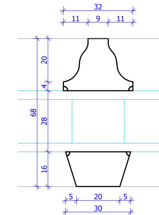
detal "B" skala 1:1
