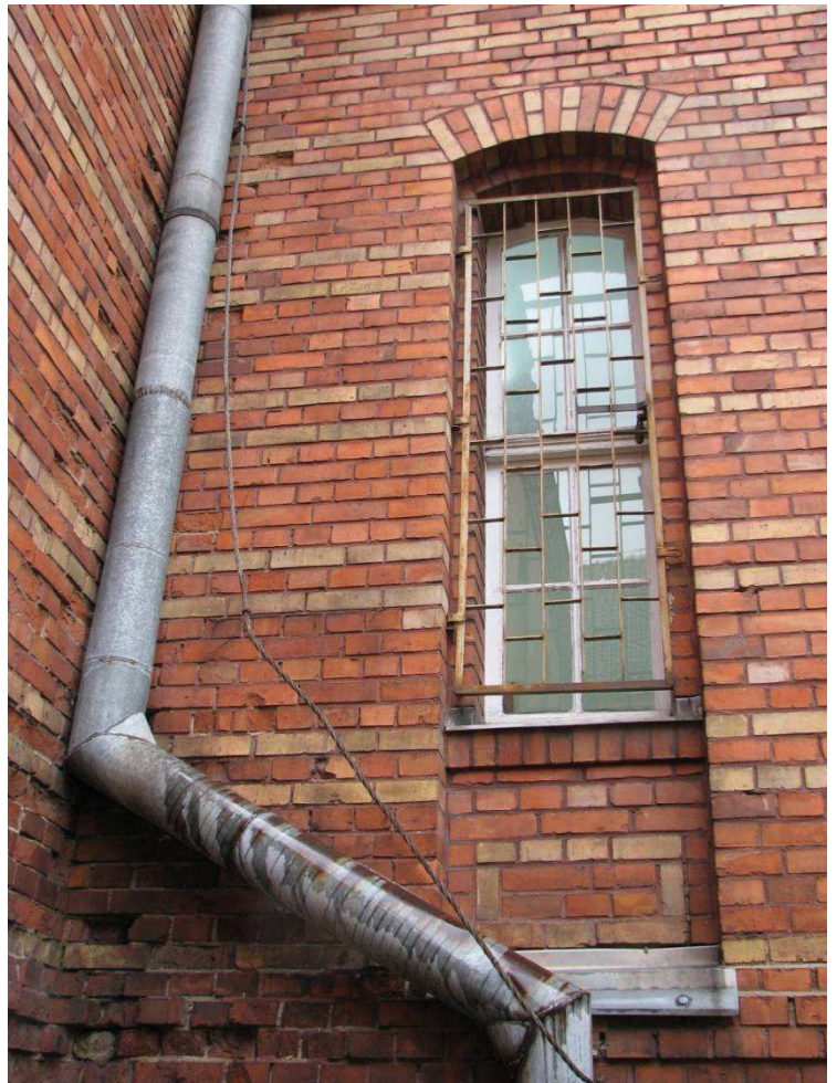
Fot. 20 Olsztyn, Kortowo, Plac Łódzki 2, stolarka okienna typ O8, widok od zewnątrz
