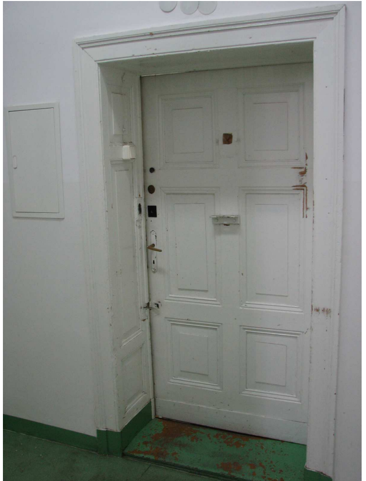
Fot. 25 Olsztyn, Kortowo, Plac Łódzki 2, stolarka drzwiowa Dz1, widok od strony klatki schodowej
