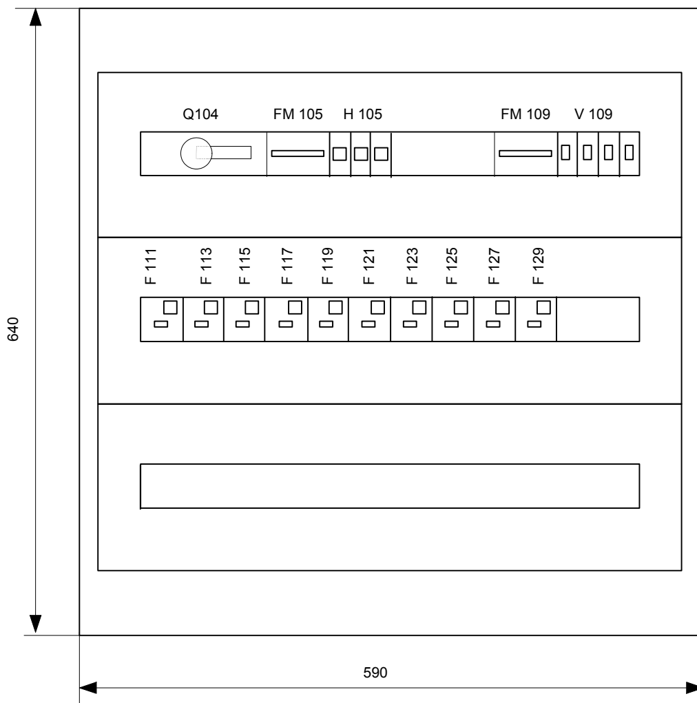
ROZDZIELNICA P/T PRAGMA F 3 x 24 IP-41 DRZWI PEŁNE - SCHNEIDER ELECTRIC
