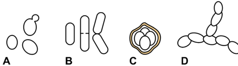
Rysunek 2 – Sposoby rozmnażania drożdży, A) przez pączkowanie np. Saccharomyces cerevisiae , B) przez podział np. Schizosaccharomyces pombe , C) worek z zarodnikami np. Saccharomyces cerevisiae , D) przez pączkowanie, formująca się pseudogrzybnią np. Candida pseudotropicalis .
