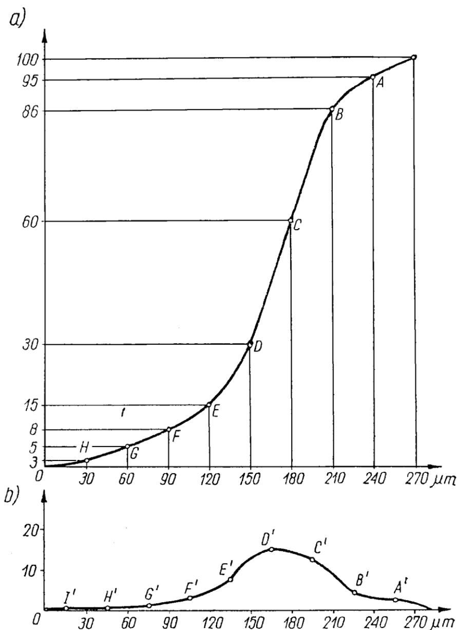
Rys. Graficzne przedstawienie granulacji młyny: a) wykres I; b) wykres II
