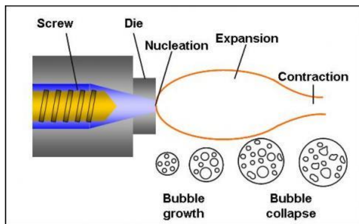
Schematyczny rysunek ekspansji ekstrudatu
