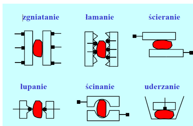
Rys. Podstawowe rodzaje sił działających na ziarno podczas rozdrabniania
